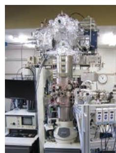
本研究グループで開発した世界初の スピン偏極透過電子顕微鏡
