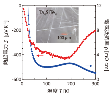
低温で高い熱電変換性能を示すTa 4 SiTe 4
