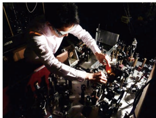
分光実験
