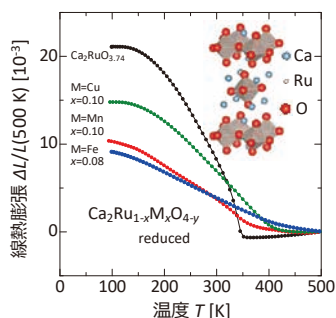
Ca 2 RuO 4 系巨大負熱膨張材料と負熱膨張の増強機構
