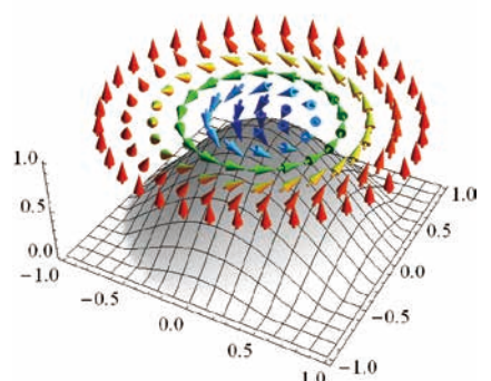
磁気スキルミオンとそれにより作られる創発磁場
