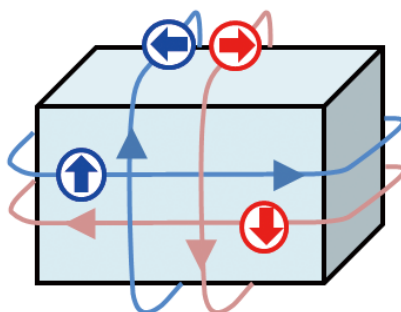
トポロジカル絶縁体の表面状態
