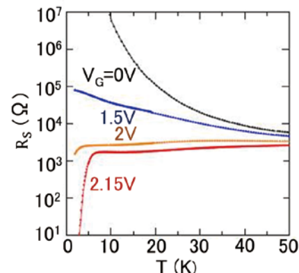
電界誘起超伝導
