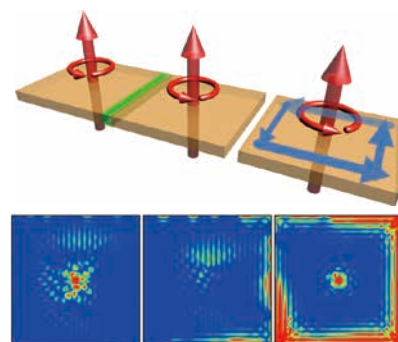
超伝導中のマヨラナフェルミオン
