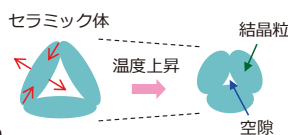
Ca 2 RuO 4 系巨大負熱膨張材料と負熱膨張の増強機構
