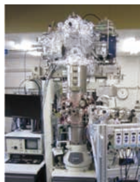
本研究グループで開発した世界初のスピン偏極透過電子顕微鏡
