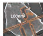
トポロジカル絶縁体単結晶上に形成したジョセフソン接合
