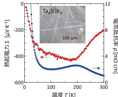
低温で高い熱電変換性能を示すTa 4 SiTe 4
