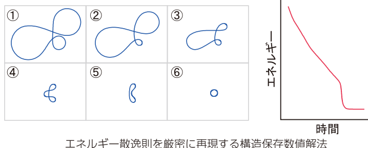
エネルギー散逸則を厳密に再現する構造保存数値解法
