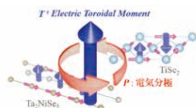
励起子絶縁体中の電気トロイダルモーメント
