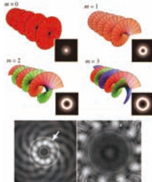
電子顕微鏡をもちいて生成した角運動量をもつ電子波
