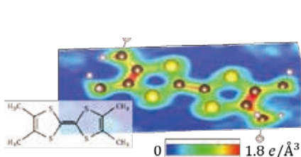
結晶中の分子軌道の直接観測
