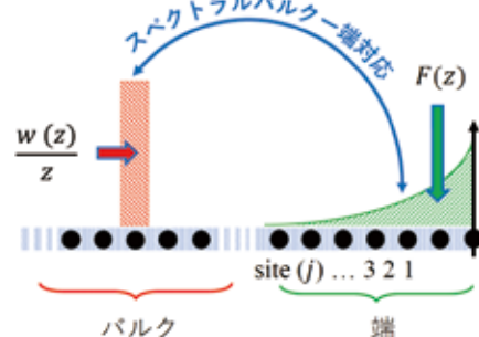
スペクトラルバルク-端対応の概念図
