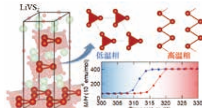
軌道電子に支配される奇妙な金属分子相
