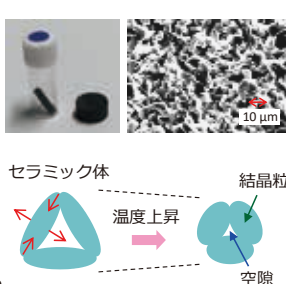
Ca 2 RuO 4 系巨大負熱膨張材料と負熱膨張の増強機構
